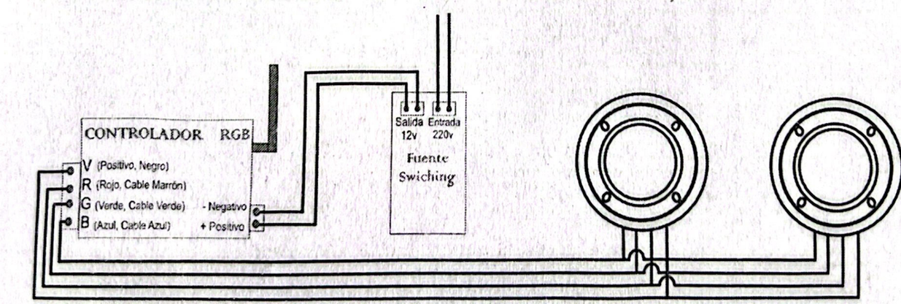
CONEXIÓN LED COLOR RGB
